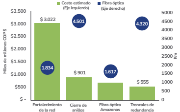
Figura 1-34. Desagregación de la inversión total en fibra óptica vs km de instalación
