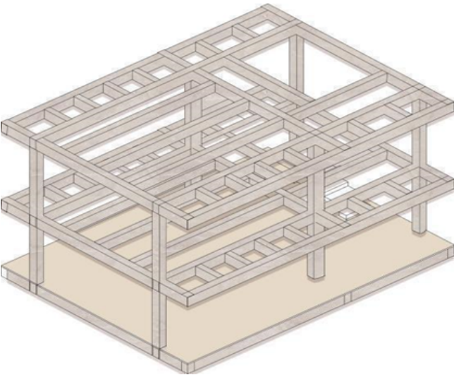
Vivienda en concreto reforzado según la norma NSR10 – estructura mínima.
