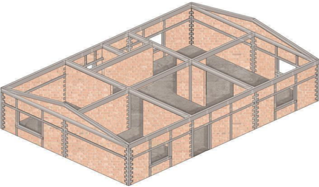
Vivienda en mampostería estructural según la norma NSR10 – estructura mínima.
