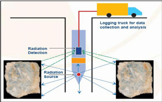
Figura 8. Perfilaje de pozos con uso de fuentes radiactivas
