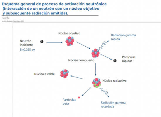
Figura 8. Esquema general de proceso de activación neutrónica (interacción de un neutrón con un núcleo objetivo y subsecuente radiación emitida).
