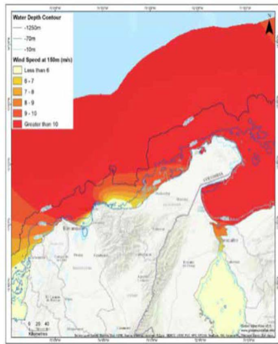
Velocidades del viento a 150 m con profundidades de referencia 10,7, 1250 m
