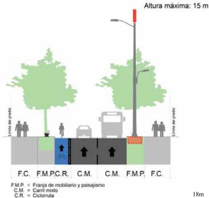
FIGURA 7-38. Altura máxima en postes localizados sobre andén
