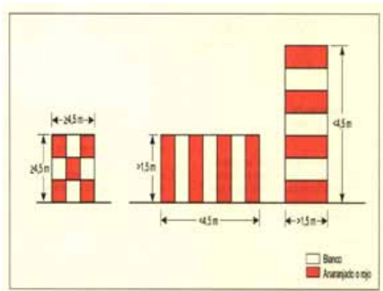
FIGURA 2-1. Configuración básica del señalamiento de obstáculos
