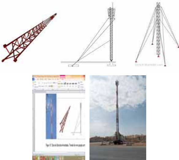
FIGURA 6-4. Estructuras de soporte arriostradas
