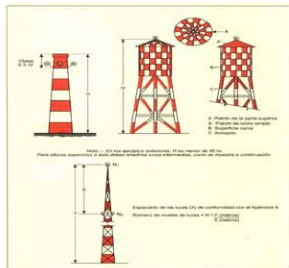
FIGURA 2-2. Señalamiento en estructuras elevadas.
