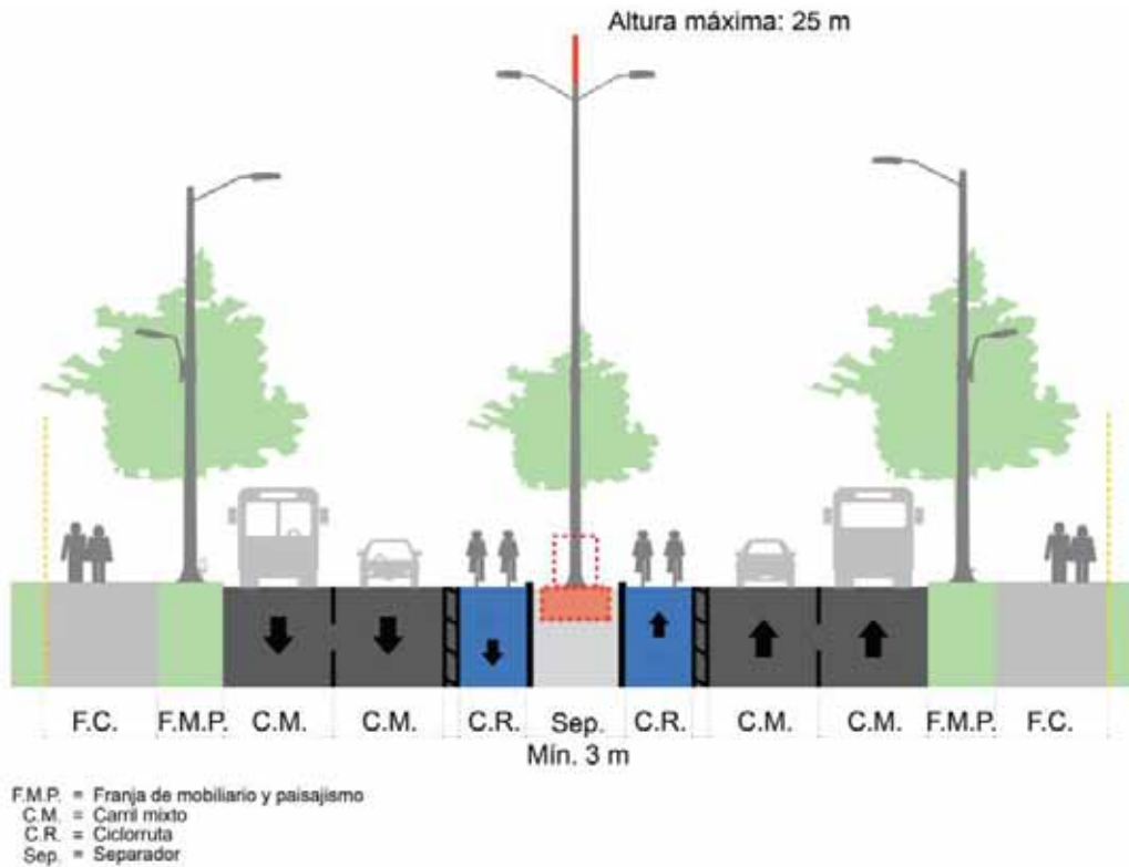
FIGURA 7-39. Altura máxima en postes localizados sobre separador con ancho \geq 3\text{m}
