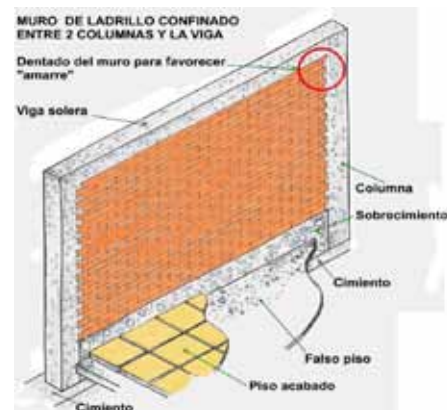
FIGURA 1-5. Cerramiento en mampostería confinada
