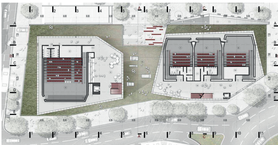
Ilustración 10_Planta generales Cinemateca Distrital _ Fuente: Colectivo 720
