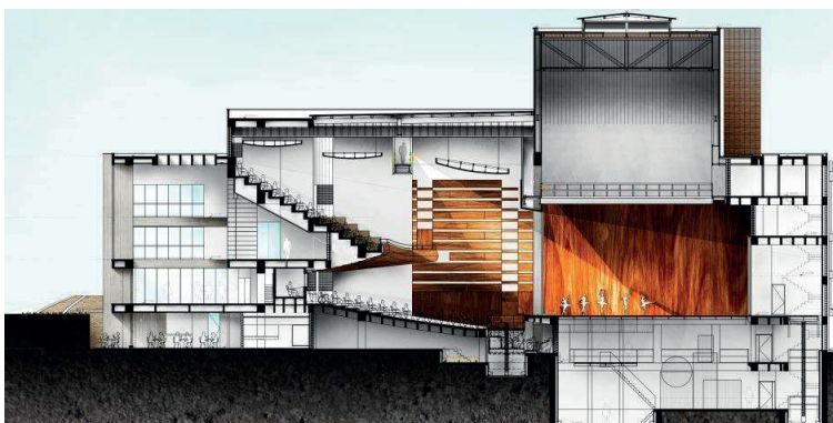
Ilustración 5_ Corte general teatro El Ensueño _ Ciudadela el ensueño_ Bogotá D.C.
