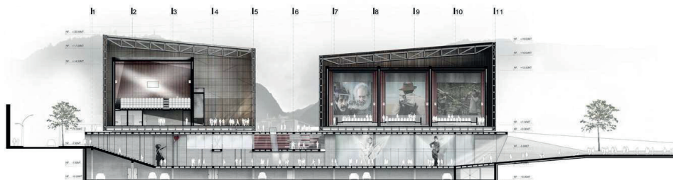
Ilustración 9_Corte general Cinemateca Distrital _ Fuente: Colectivo 720
