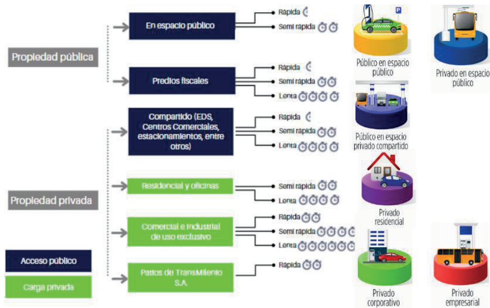
Gráfica 15 Tipos de infraestructura de recarga de vehículos eléctricos
