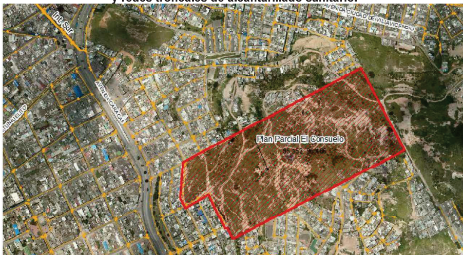
Ilustración 7. Localización del Plan Parcial El Consuelo y redes troncales de alcantarillado sanitario.
