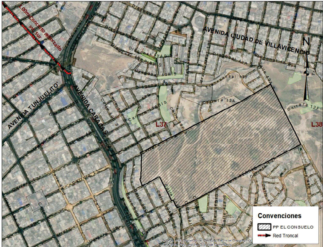
Ilustración 3. Red Troncal existente de Alcantarillado Sanitario
