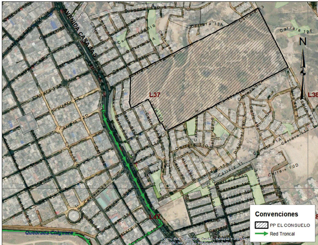
Ilustración 5. Red Troncal existente de Alcantarillado Pluvial
