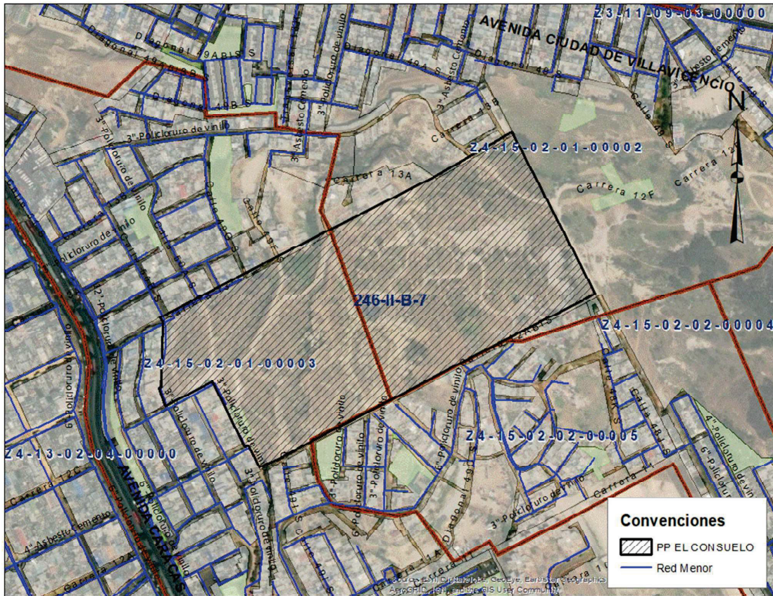
Ilustración 2. Redes menores de Acueducto existentes
