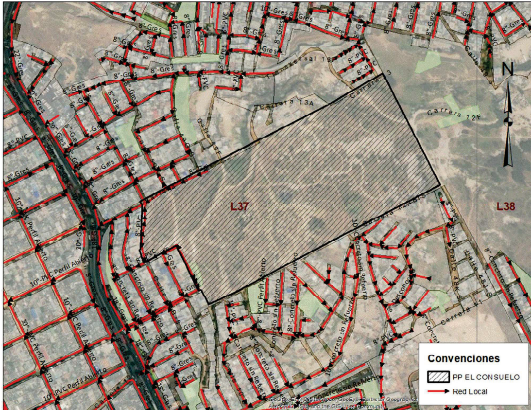
Ilustración 4. Redes Locales existentes de Alcantarillado Sanitario
