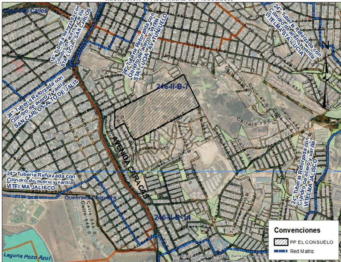
Ilustración 1. Red Matriz de Acueducto
