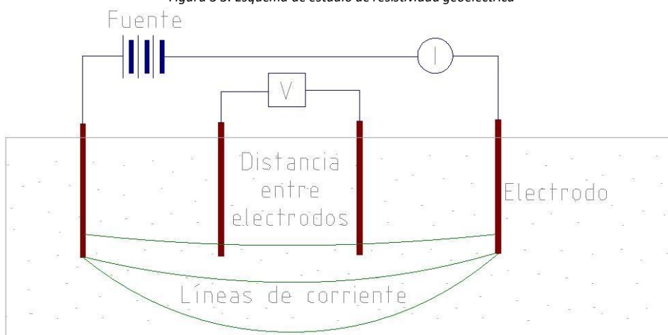
Figura 3 3. Esquema de estudio de resistividad geoelectrica
