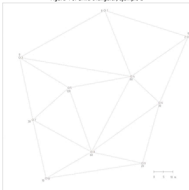
Figura 4 6. Grilla triangular, Ejemplo 1
