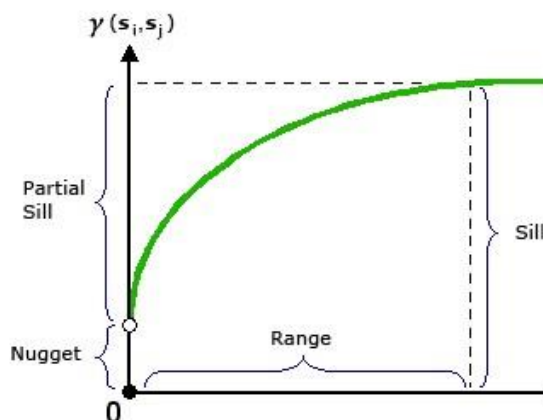
Figura 4 12. componentes de rango, meseta y nugget
