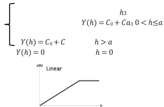
Figura 4 17. modelo de semivarianza lineal
