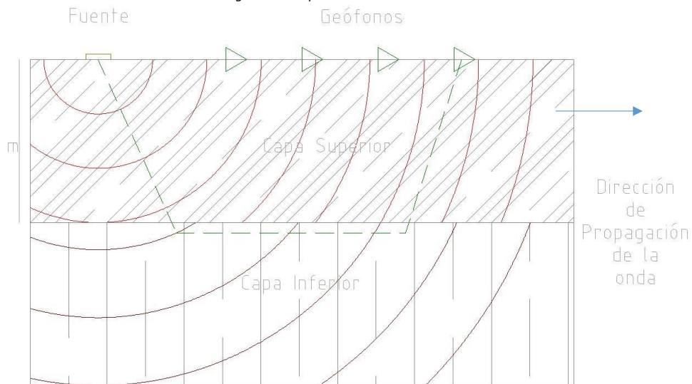
Figura 3 1. Esquema de estudio sísmico.
