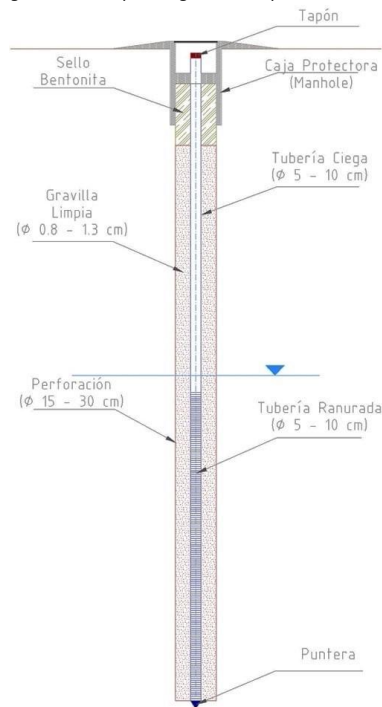
Figura 4 20. esquema general de pozo de monitoreo
