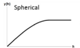
Figura 4 14. modelo de semivarianza circular
