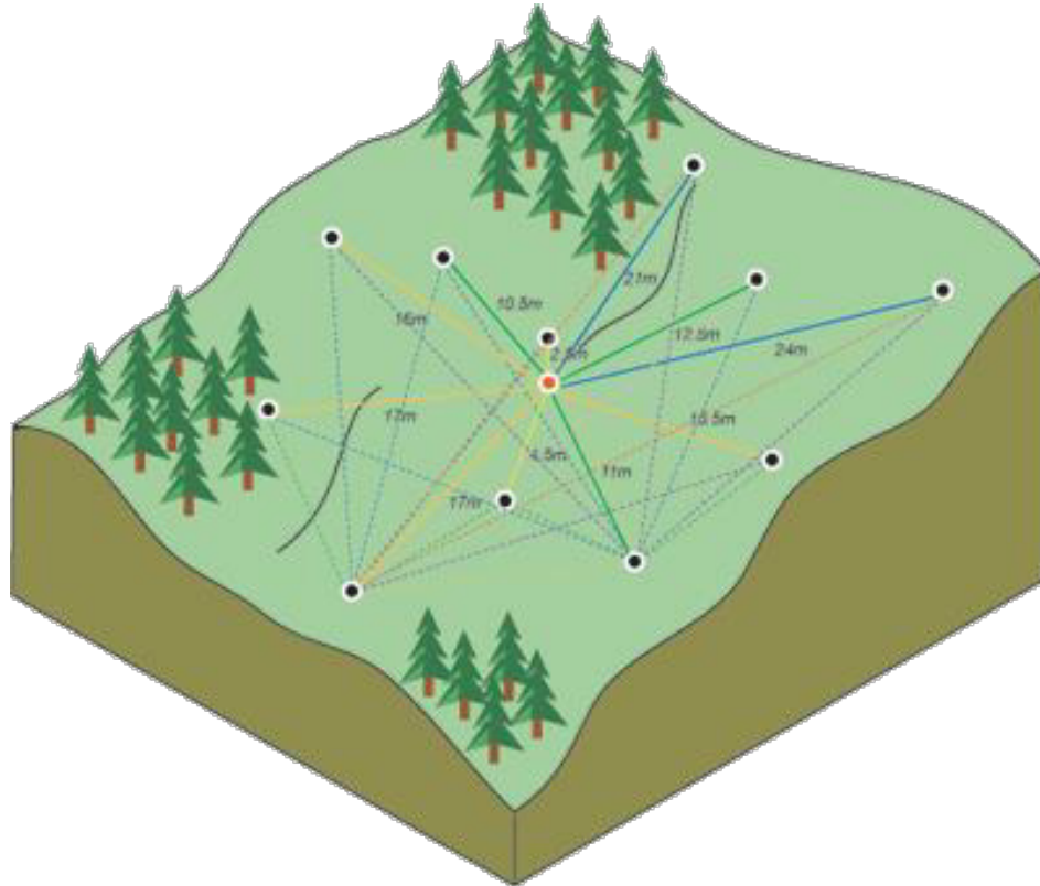
Figura 4 10. Cálculo de la diferencia cuadrada entre las ubicaciones asociadas
