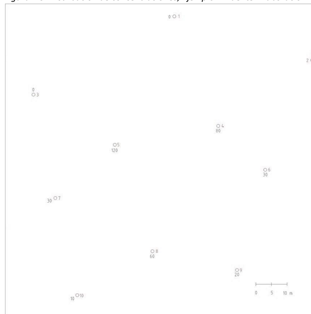
Figura 4 5. Distribución de concentraciones, Ejemplo 1. Fuente: Elaboración Propia
