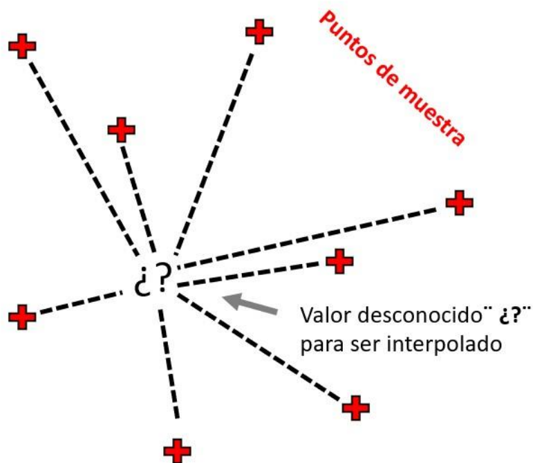
Figura 4 18. Interpolación Distancia Inversa Ponderada basada en la distancia del punto de muestra ponderada
