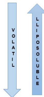
Ilustración 1: Grafica de relación del grado de clorinación de los PCB con relación a su lipofilidad.
