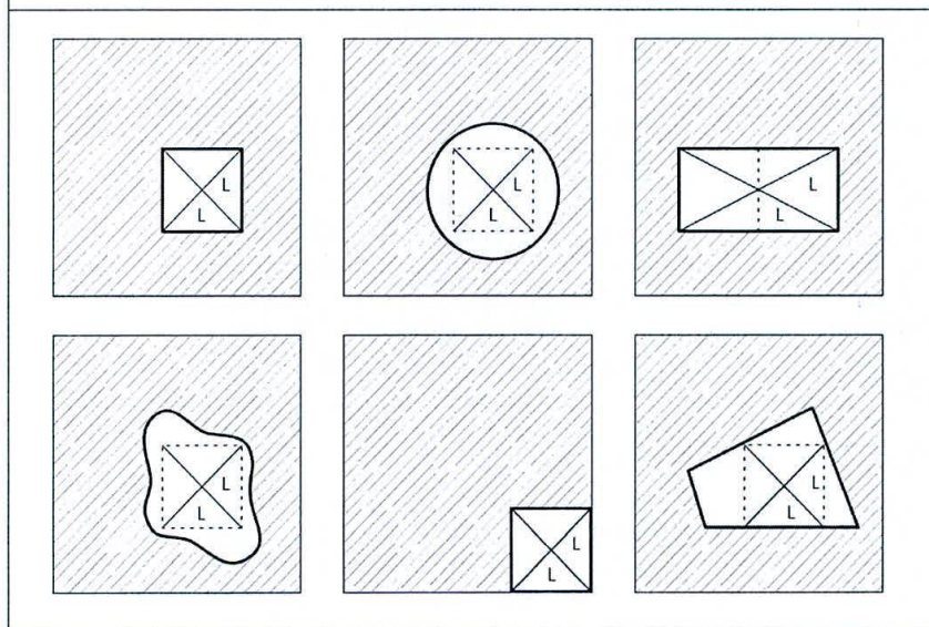
Ilustración 16. SECCIÓN 1.12.b. Dimensionamiento de patios. Ejemplos de configuración.
