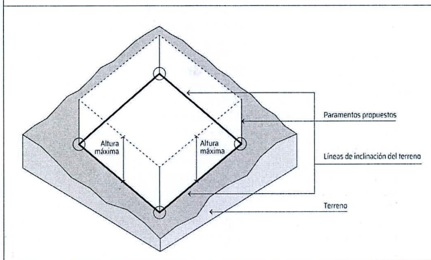
Ilustración 04. SECCIÓN 1.1. CONCEPTOS Y DEFINICIONES. Línea de inclinación del terreno.
