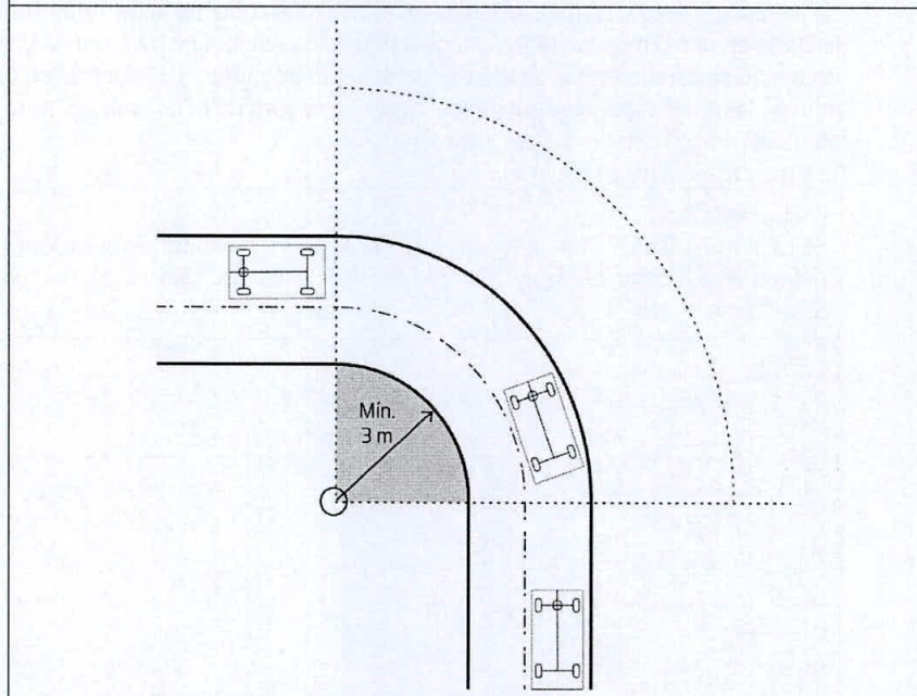
Ilustración 24. SECCIÓN 1.23.k. Dimensiones de circulación y áreas de maniobra para automóviles, camionetas y camperos - Radio mínimo. SECCIÓN 1.23.m. Rampas vehiculares.
