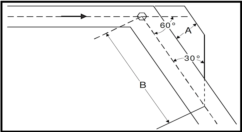
Figura 15-3.– Caso de dos tramos de ruta que se cortan a un ángulo de 60° en la intersección de dos radiales VOR, más allá del punto en que debe ensancharse el espacio aéreo protegido con objeto de atenerse a lo prescrito en 3.3.
