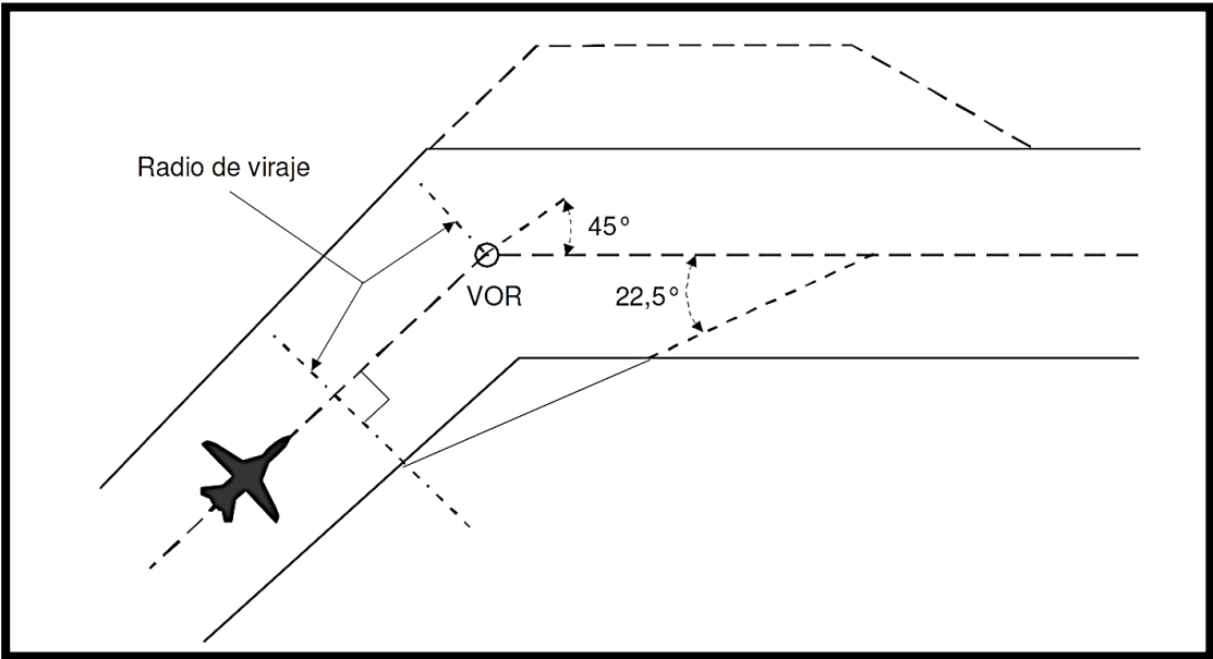
Figura 15-5.– Método para construir el espacio aéreo protegido adicional requerido en la parte interior de los virajes de 90° o menos.
