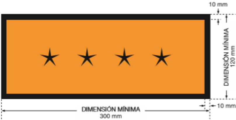
Figura 7:Rótulo para indicar por separado el número de las Naciones Unidas. El color de fondo del rótulo será naranja y los bordes y el número de las Naciones Unidas serán negros. El símbolo “****” indica el espacio en el que deberá insertarse el número de las Naciones Unidas apropiado para los materiales radiactivos de que se trate, según se especifica en el Cuadro 1.
