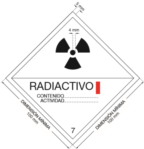
Figura 2: Etiqueta para la categoría I-BLANCA. La anchura mínima de la línea dentro del borde
