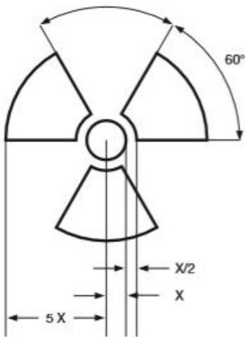
Figura 1: Símbolo fundamental: un trébol cuyas proporciones están basadas en un círculo central de radio X. La dimensión mínima admisible de X será de 4 ms.
