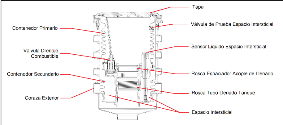
Ilustración 8. Ejemplo de Contenedor de Derrames de doble pared
