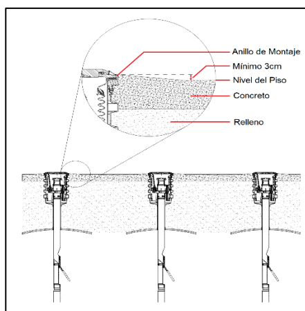
Ilustración 4. Ejemplo boca de llenado con Contenedor de Derrames que sobresale para evitar el ingreso de agua
