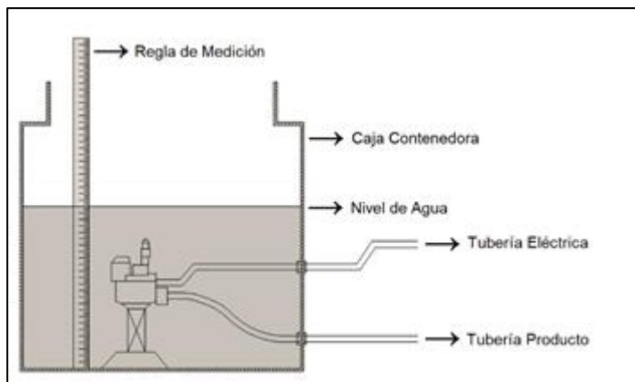
Ilustración 12. Ejemplo de Prueba de Estanqueidad en la caja contenedora
