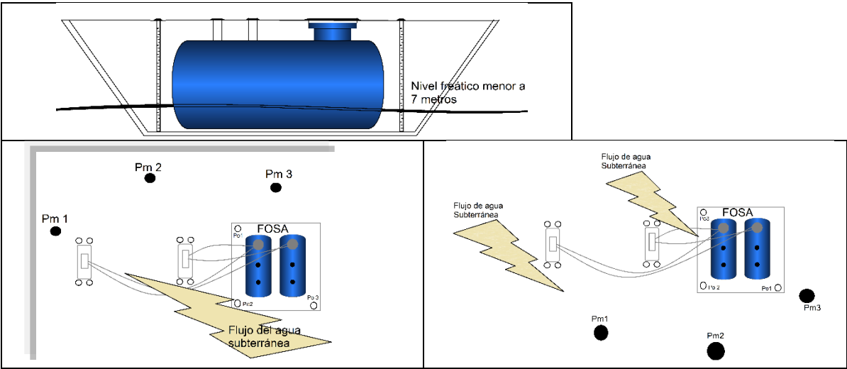
Ilustración 7. Ejemplo ubicación Pozo de Monitoreo (Pm)
