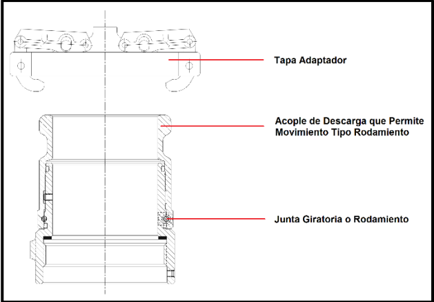
Ilustración 9. Ejemplo de acople de descarga
