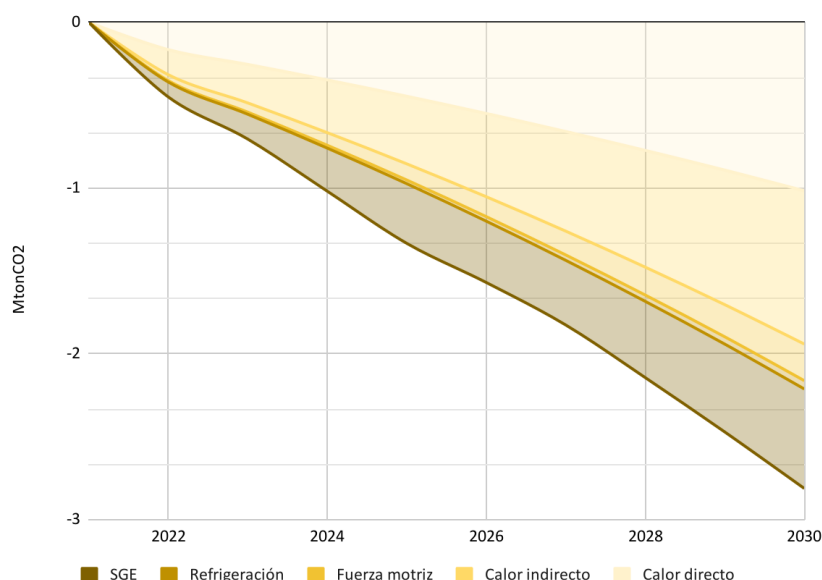
Gráfica 22. Reducción estimada de emisiones de las medidas de eficiencia energética en el sector industrial en el PAI-PROURE
