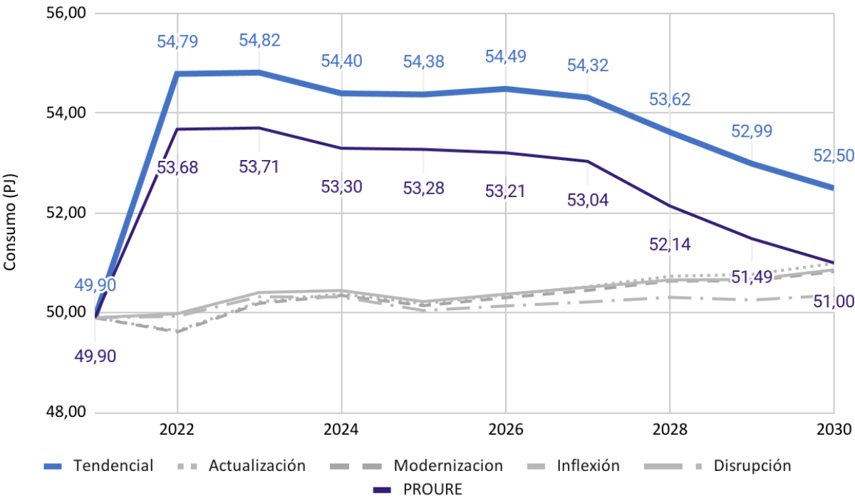
Gráfica 36. Comparación de escenarios de consumo energético para el sector minero
