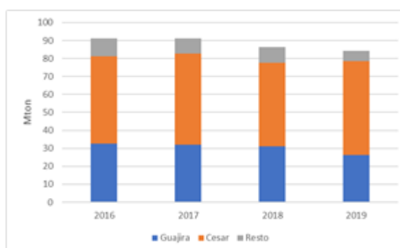
Producción Nacional de Carbón
