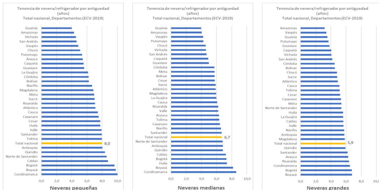
Gráfico 43. Edad promedio de las neveras por departamento
