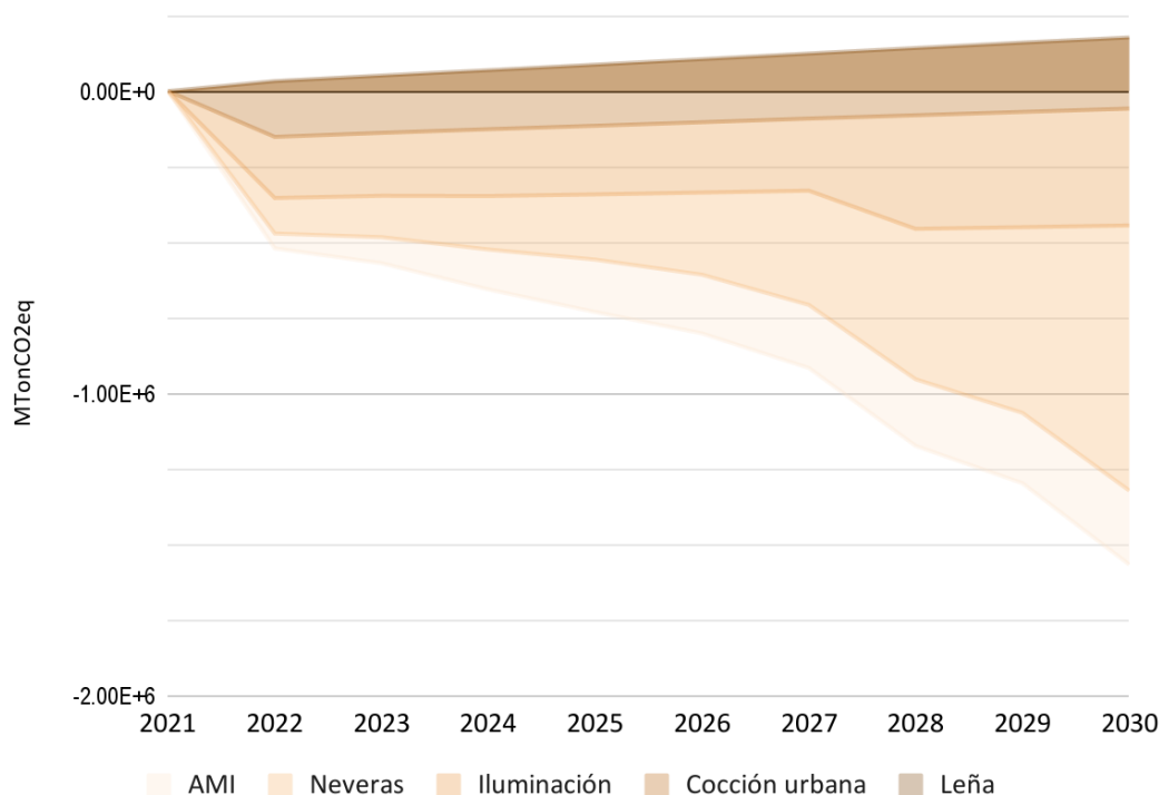
Gráfica 12. Reducción estimada de emisiones de las medidas de eficiencia energética en el sector residencial en el PAI-PROURE
