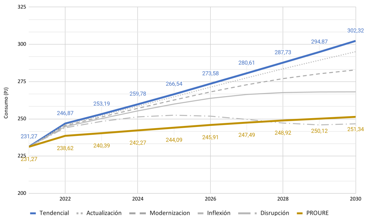
Gráfica 20. Comparación de escenarios de consumo energético para el sector industrial.
