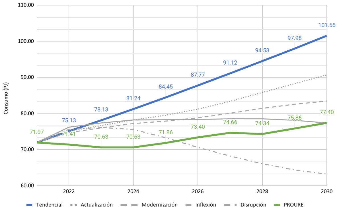
Gráfica 24. Comparación de escenarios de consumo energético para el sector terciario.
