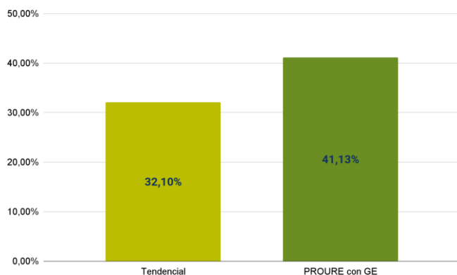
Gráfica 52. Porcentaje de energía útil sobre energía final
