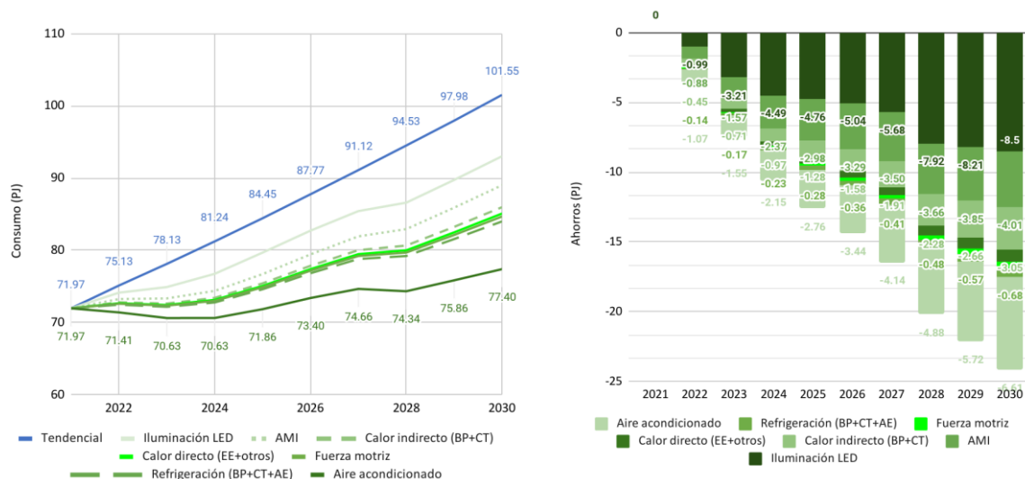
Gráfica 25. Reducción de demanda esperada de las medidas de eficiencia energética en el sector terciario en el PAI-PROURE
