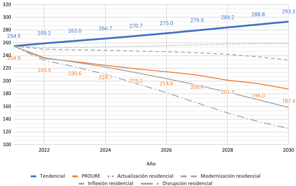
Gráfica 10. Comparación de escenarios de consumo energético para el sector residencial.
