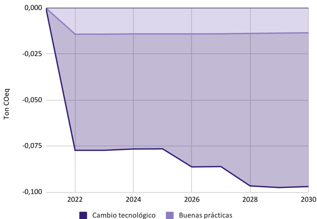
Gráfica 38. Reducción estimada de emisiones de las medidas de eficiencia energética en el sector minero en el PAI-PROURE
