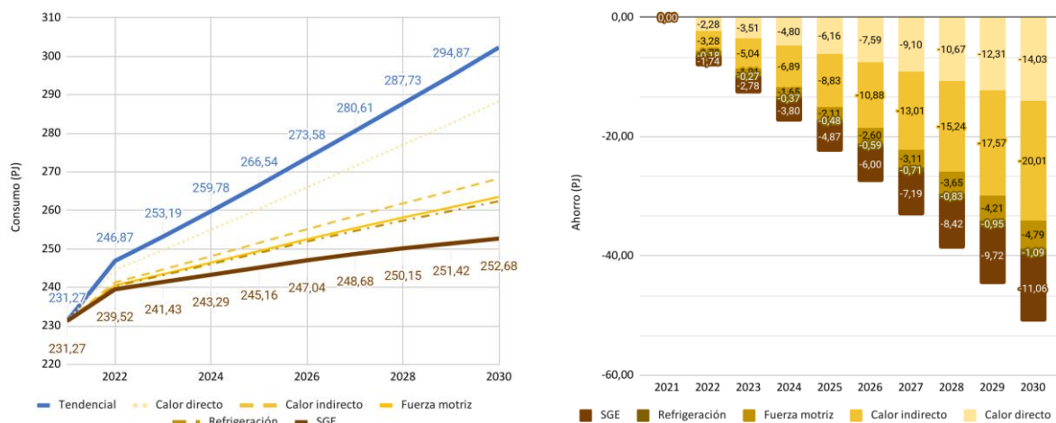
Gráfica 21. Reducción de demanda esperada de las medidas de eficiencia energética en el sector industrial en el PAI-PROURE
