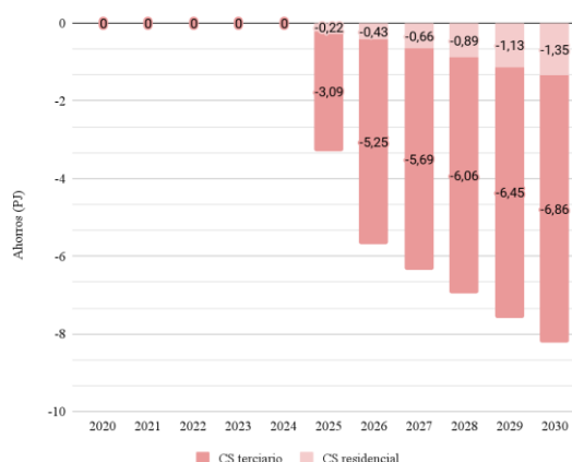
Gráfica 40. Reducción de demanda esperada de las medidas de eficiencia energética de construcción sostenible.
