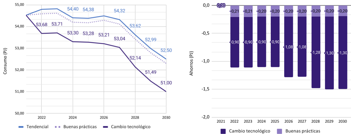
Gráfica 37. Simulación de los ahorros energéticos en el sector minero por la adopción de las medidas analizadas.
