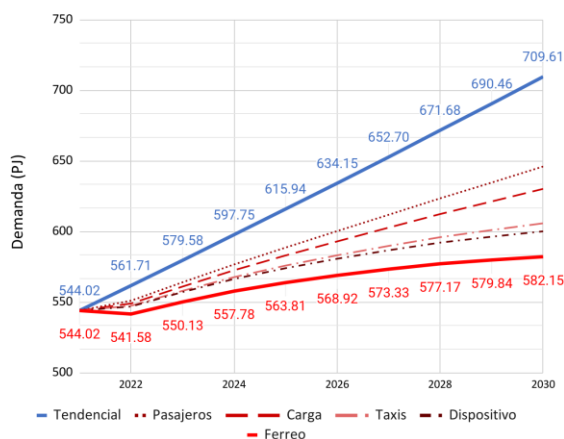
Gráfica 16. Reducción de demanda esperada de las medidas de eficiencia energética en el sector transporte en el PAI-PROURE
