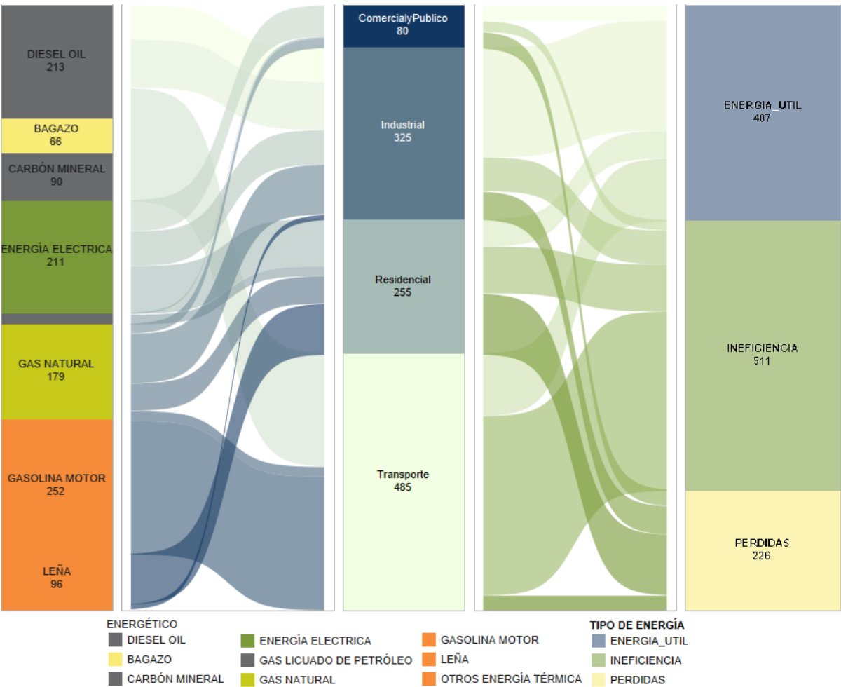
Gráfica 1. Balance de energía útil 2019 5
