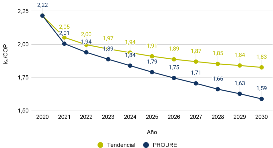
Gráfica 51. Indicador de intensidad energética (kJ/COP)
