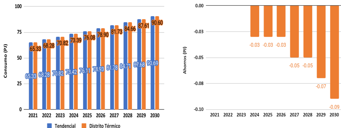
Gráfica 42. Reducción de demanda esperada de las medidas de eficiencia energética por distritos térmicos
