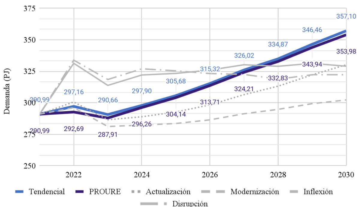
Gráfica 28. Comparación de escenarios de consumo energético para el sector termoeléctrico.
