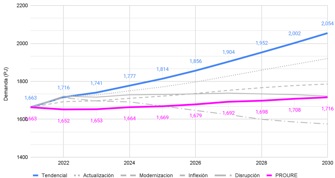
Gráfica 3. Comparación del consumo estimado para el escenario PAI-PROURE 2022-2030 frente al escenario tendencial y los del PEN 2020-2050
