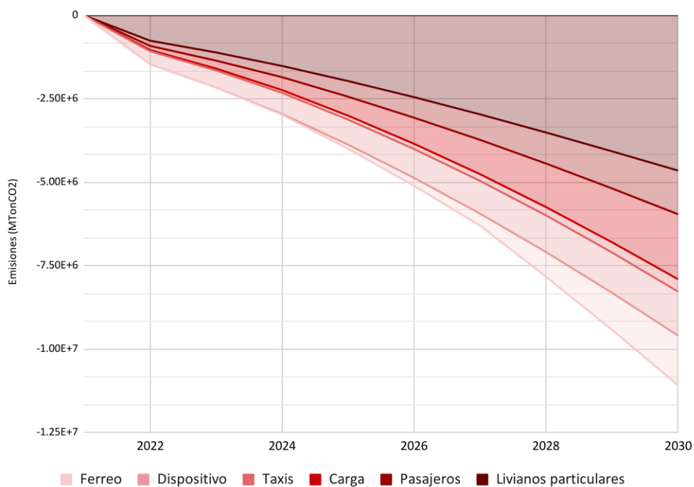
Gráfica 18. Reducción estimada de emisiones de las medidas de eficiencia energética en el sector transporte en el PAI-PROURE
