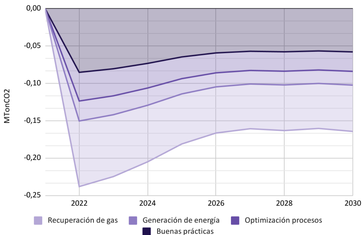
Gráfica 34. Reducción estimada de emisiones de las medidas de eficiencia energética en el sector hidrocarburos en el PAI-PROURE
