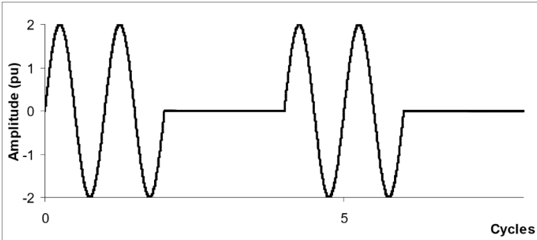
b) Corriente de prueba de subarmónicos, 2 ciclos encendidos, 2 ciclos apagada
