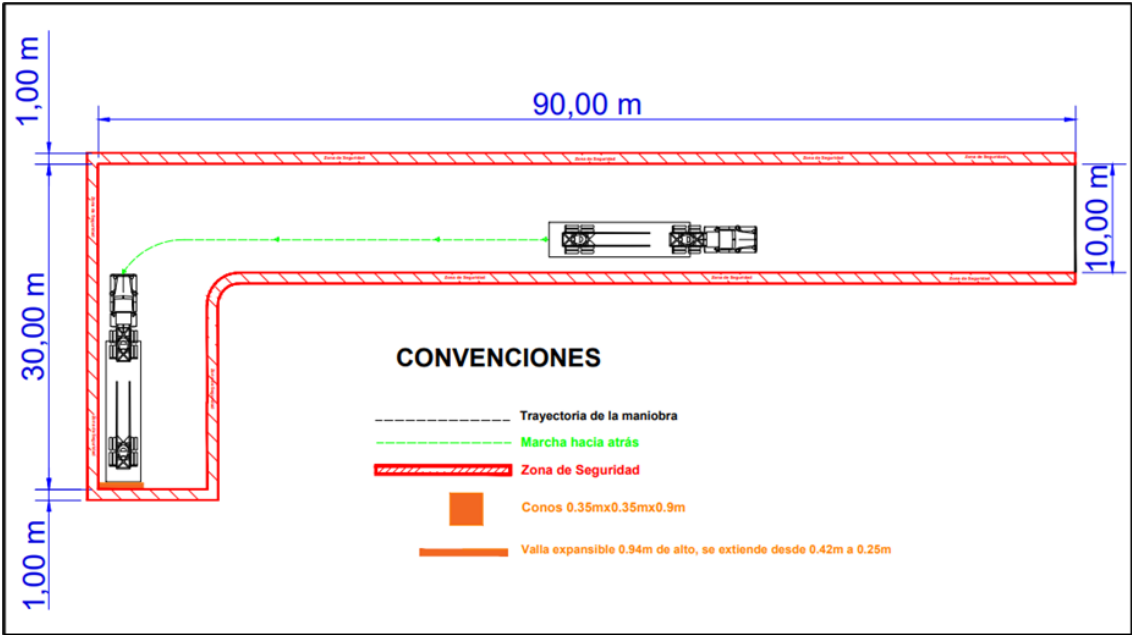
Ilustración 20. Maniobra de marcha atrás en recta y curva para categorías B3 y C3
