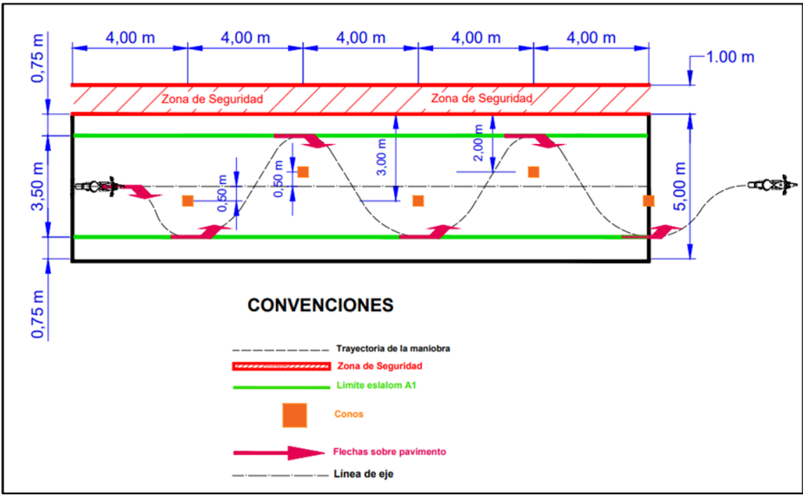
Ilustración 3. Maniobra de esalon a baja velocidad para categorías A1 y A2
