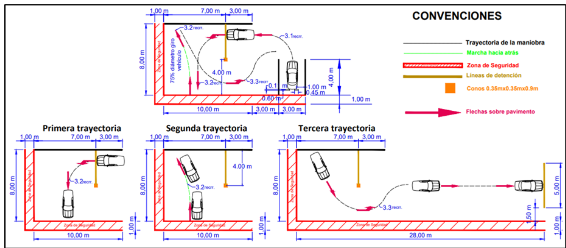
Ilustración 12. Maniobra de cambio de sentido de la marcha en espacio limitado para categorías B1 y C1
