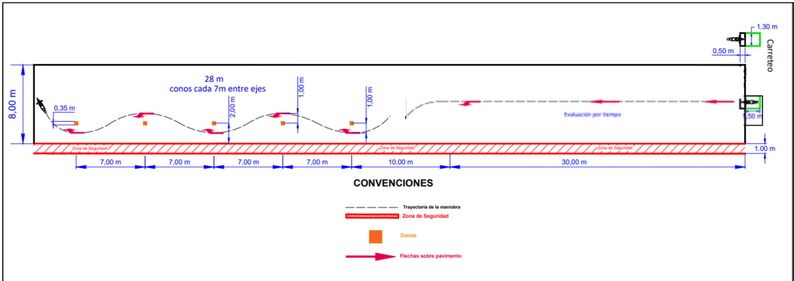
Ilustración 5. Maniobra de Eslalon a alta velocidad y Maniobra 4.1. Interacción con señales de tránsito verticales- Giro en U para categorías A1 y A2
