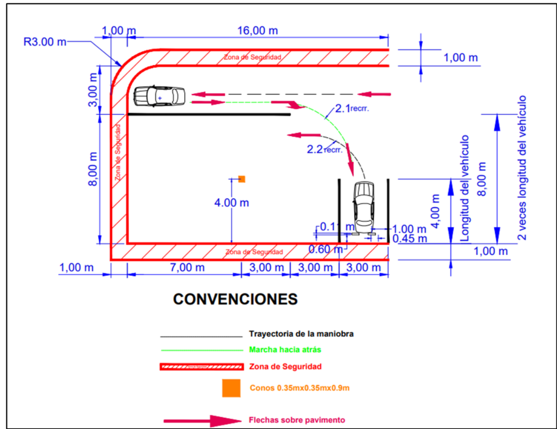
Ilustración 11. Maniobra de reversa en curva para estacionamiento en perpendicular para categorías B1 y C1
