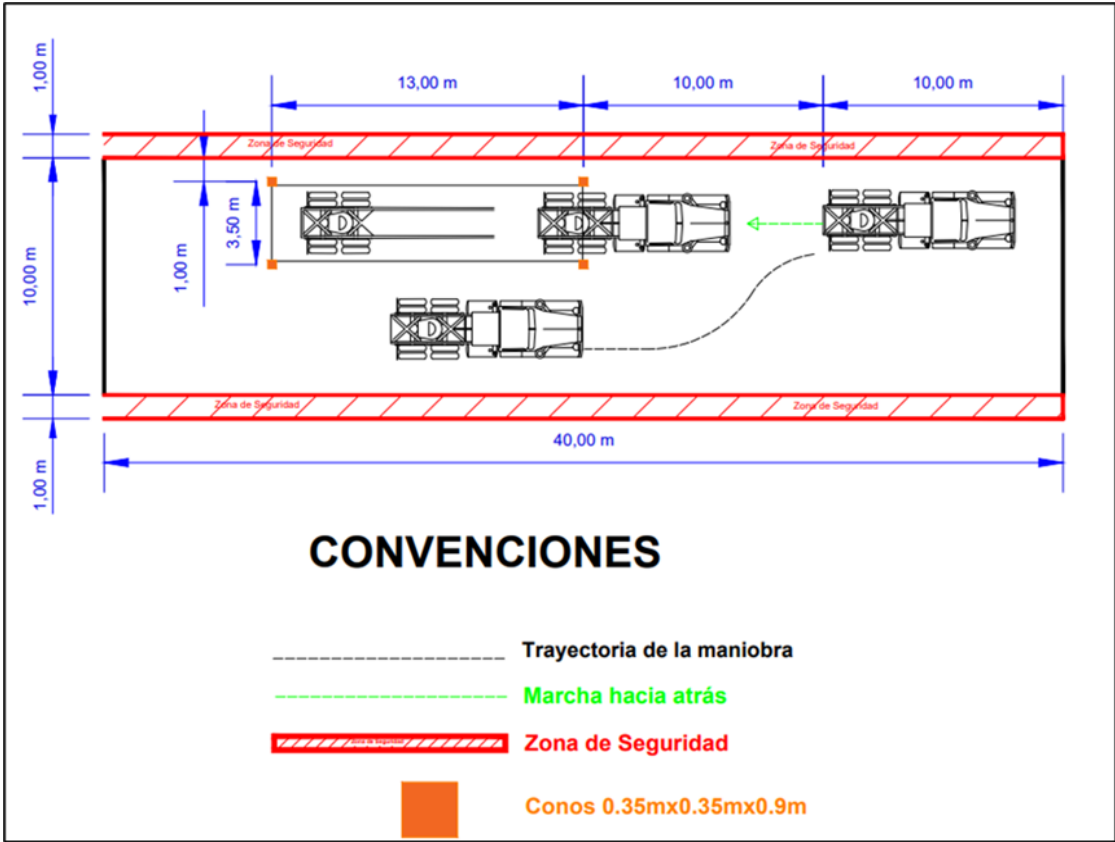
Ilustración 19. Maniobra de acoplamiento del semirremolque para categorías B3 y C3
