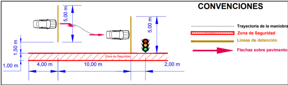
Ilustración 14. Interacción con señal semafórica para categorías B1 y C1.
