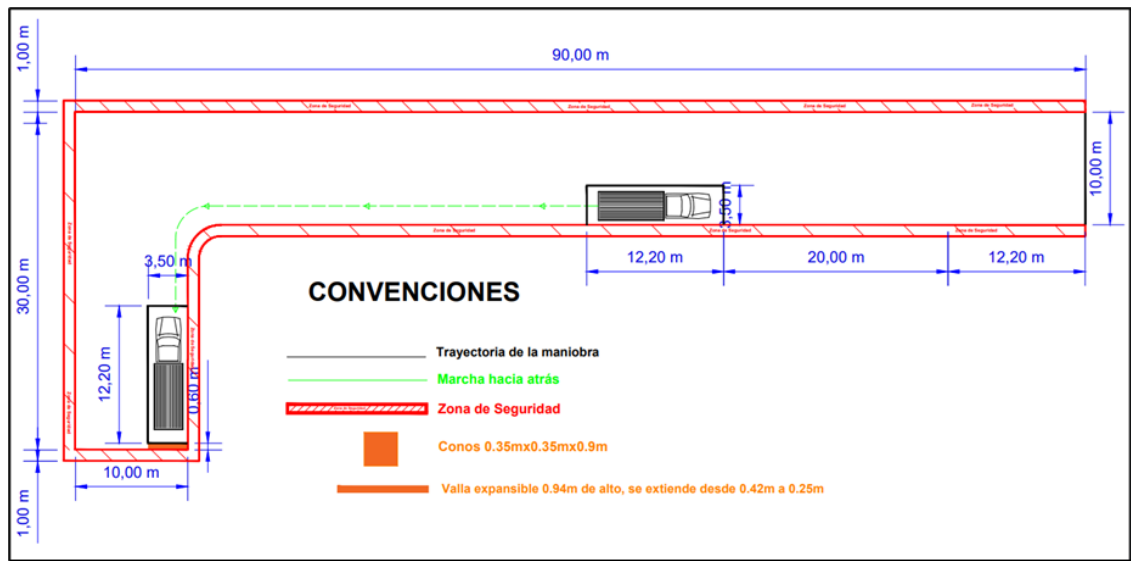
Ilustración 18. Maniobra de marcha atrás en recta y curva para categorías B2 y C2
