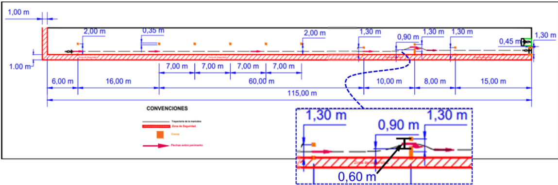
Ilustración 7. Maniobra de sorteo de un obstáculo a velocidad de 30 km/h y frenado de emergencia para categorías A1 y A2
