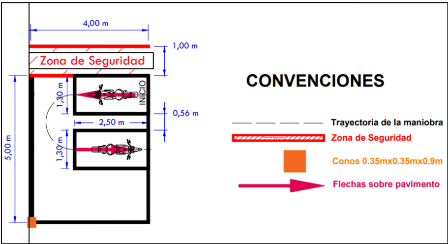
Ilustración 1. Maniobra de carreteo para categorías A1 y A2
