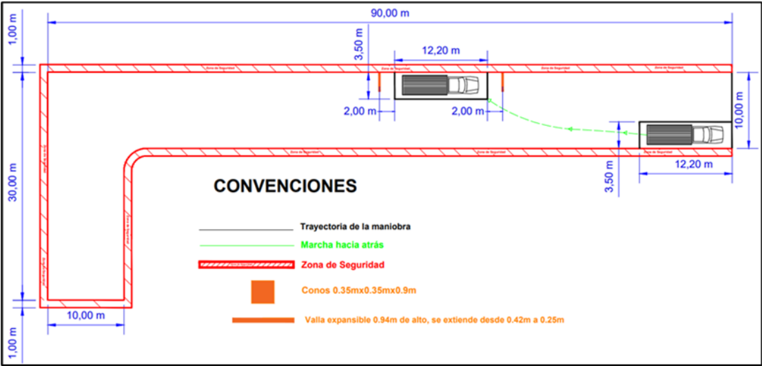
Ilustración 17. Maniobra de estacionamiento en línea para categorías B2 y C2
