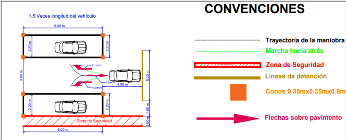
Ilustración 13. Maniobra de estacionamiento en línea para para categorías B1 y C1
