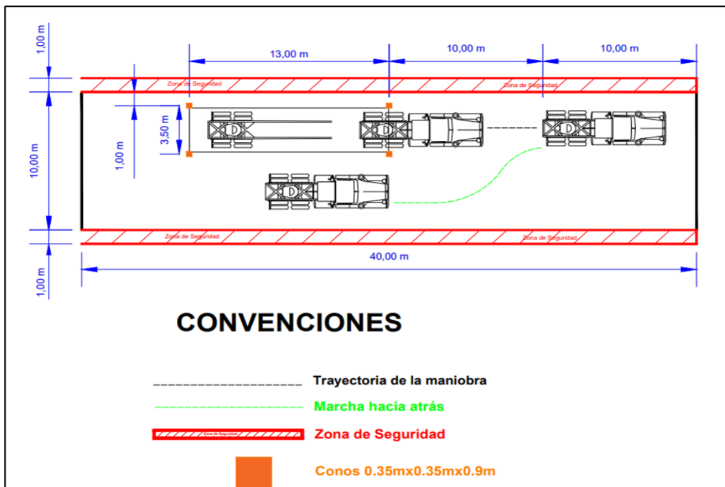
Ilustración 21. Maniobra de desacoplamiento del semirremolque
