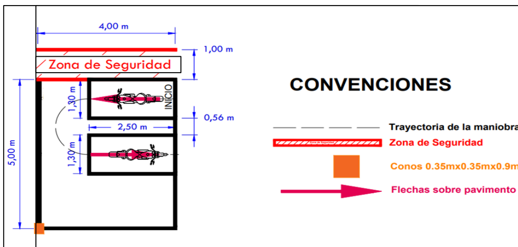
Ilustración 1. Maniobra de carreteo para categorías A1 y A2
